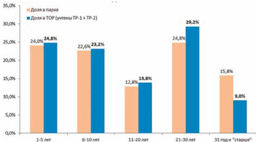
Рис. 5. Доли вагонов различных «возрастных групп» в ТОР в сравнении с долями в парке вагонов за первое полугодие 2015 г.
