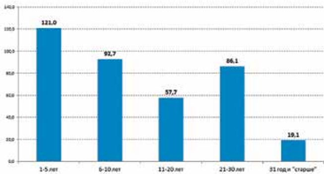
Рис. 1. Количество отцепок в ТР-2 грузовых вагонов с различным сроком службы («возрастом») за первое полугодие 2015 г., тыс. случаев
