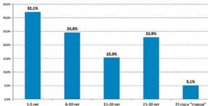
Рис. 2. Доли отцепок грузовых вагонов с различным сроком службы («возрастом») от общего количества отцепок в ТР-2 за первое полугодие 2015 г., %
