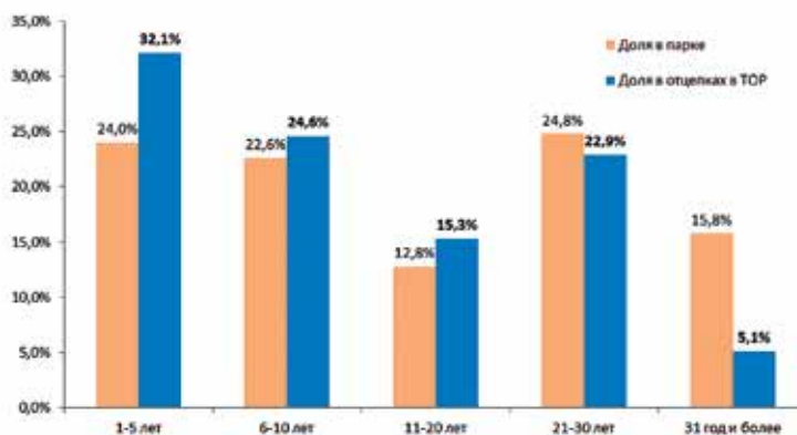
Рис.4. Доли отцепок вагонов различных «возрастных групп» в ТР-2 в сравнении с долями в эксплуатируемом парке грузовых вагонов за первое полугодие 2015 г., %
